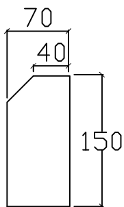
後牆尺寸
